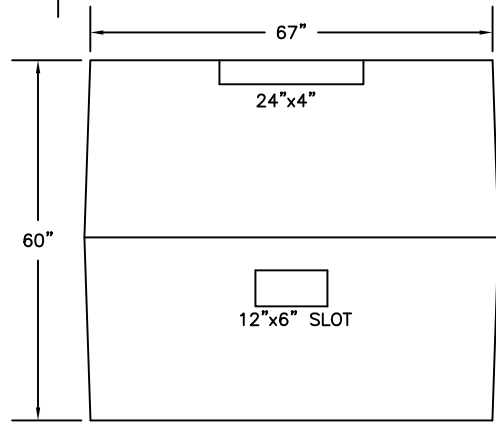
BAFFLE
